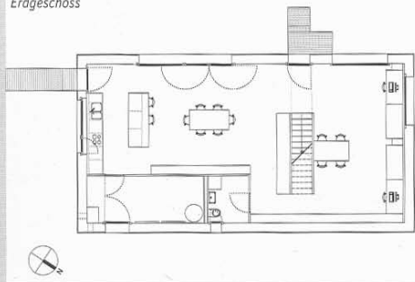
Erdgeschoss
